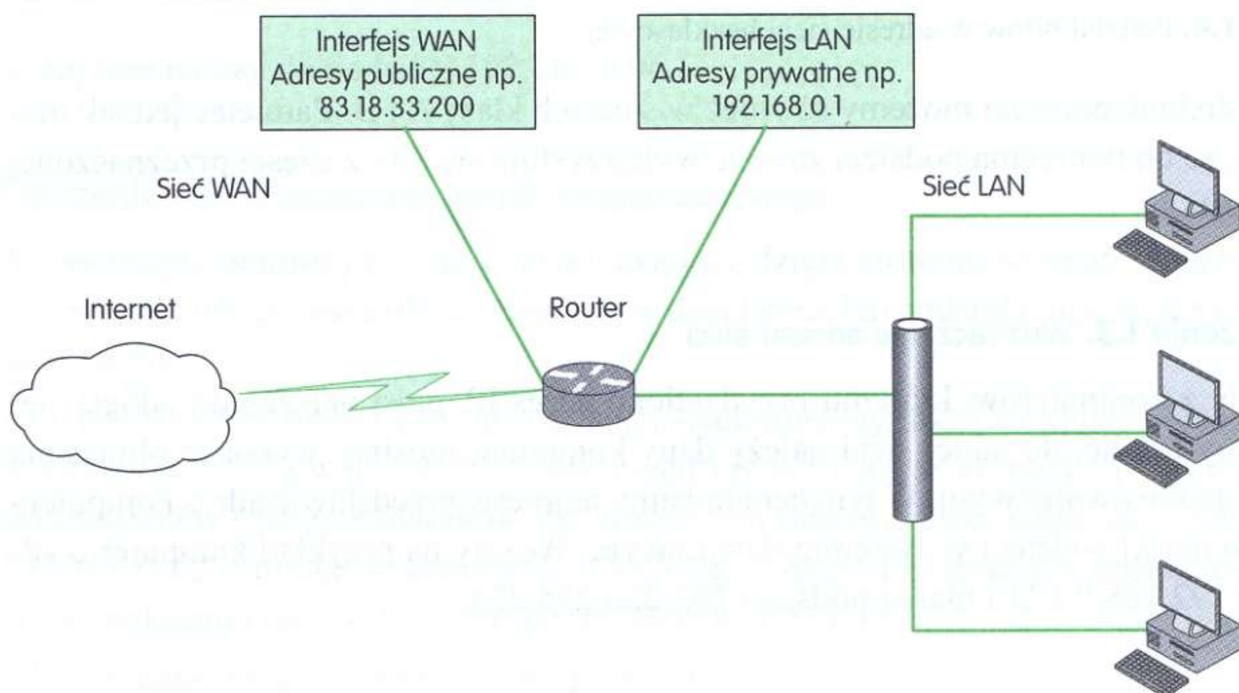
Rys. 1.7. Schemat sieci lokalnej przyłączonej do Internetu za pomocą routera
